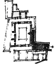
شكل ٣ استخدام المدخل المنكسر والرواشين لتحقيق الخصوصية
